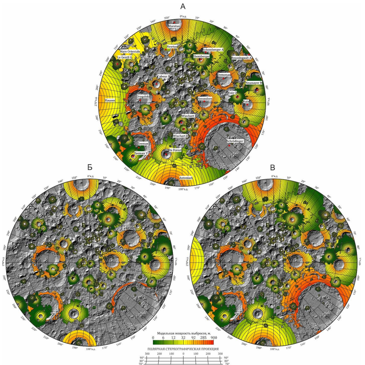
Рис. 2. Модельная мощность выбросов кратеров нектарианского - коперниковского возраста в районе южного полюса Луны. А – без учета смешения материала; В – с учетом смешения материала по Oberbeck и др. (1975); С – с учетом смешения материала по Petro и Pieters (2006).
