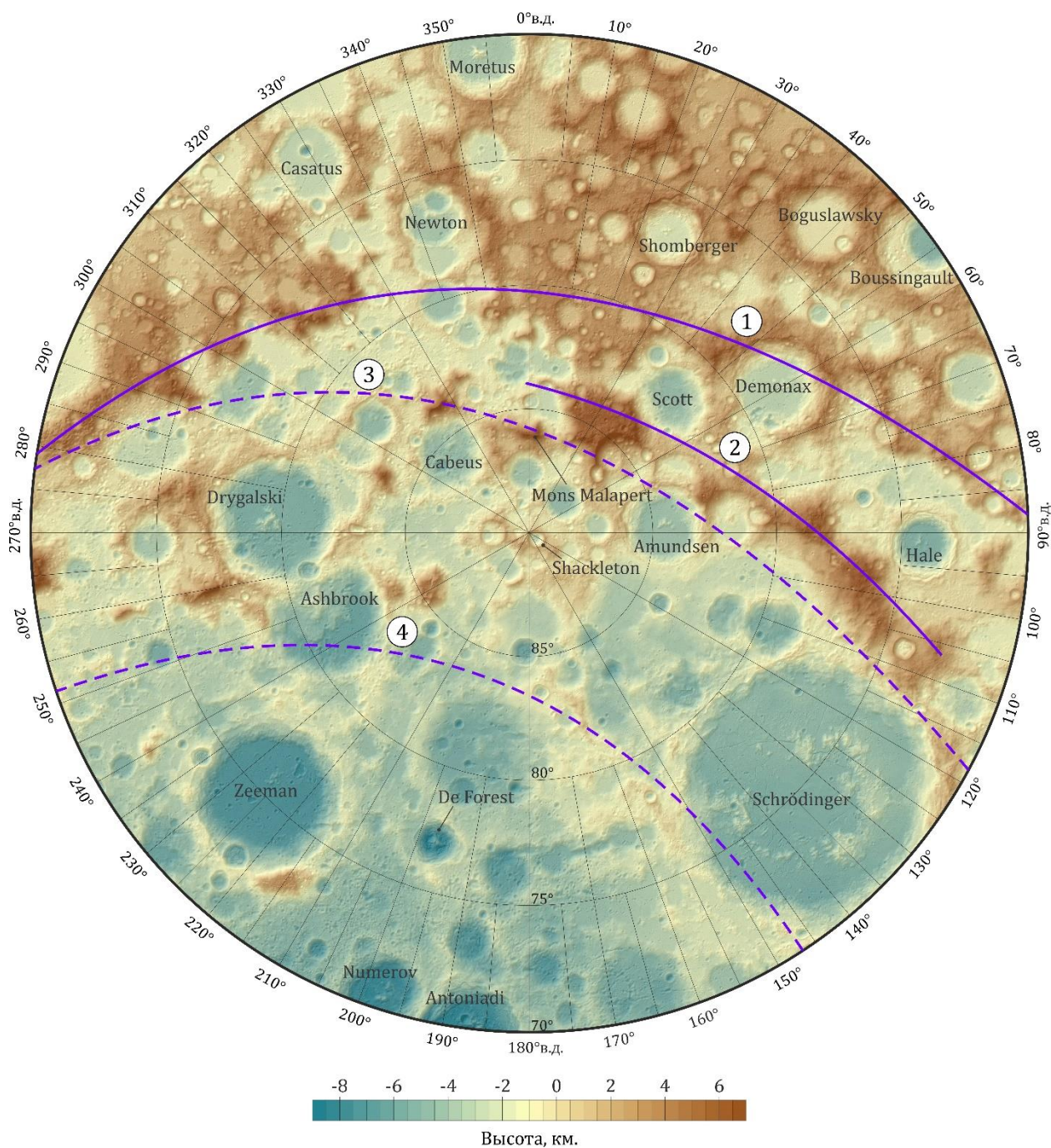
Рис. 1. Предполагаемые границы бассейна SPA: 1 - Эллипс SPA по (Wilhelms и др., 1979). 2 - массивы SPA, хорошо коррелирующие с (3) внешним эллипсом по (Garrick-Bethell и Zuber, 2009). (4) внутренний эллипс по Garrick-Bethell и Zuber, (2009).
